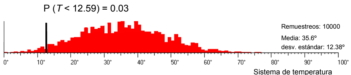
Figura 2.4. Se muestra el resultado obtenido con el software “NESTEDNESS CALCULATOR”. La rutina de Monte Carlo se realizó con 10000 aleatorizaciones (remuestreros).
